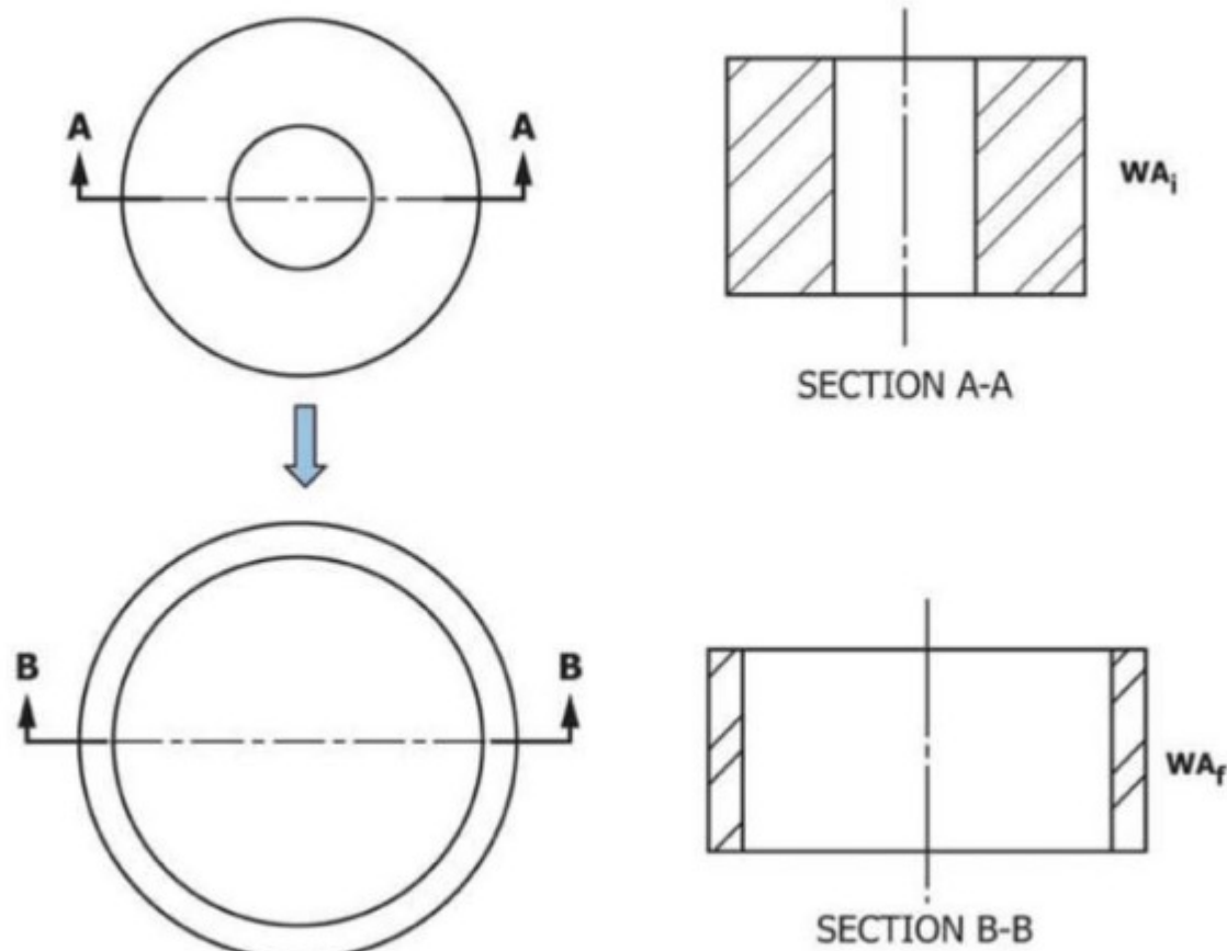
FIG. X1.4 Ring Rolling
